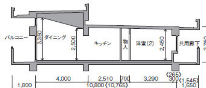
6号棟1402・1403号室、18号棟1402・1403号室 最上階住宅A-A'断面図 ※〈 〉内寸法は18号棟を表します。
