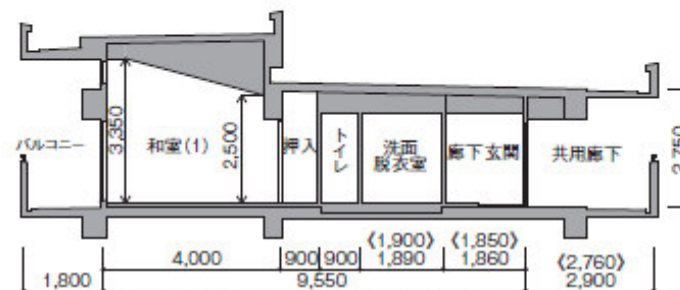
6号棟1402・1403号室、18号棟1402・1403号室 最上階住宅B-B'断面図 ※〈 〉内寸法は18号棟を表します。
