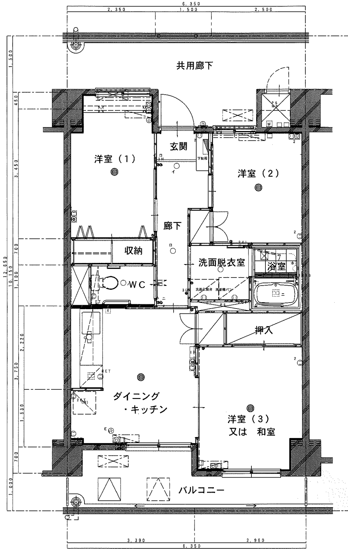
3DK 平面図
