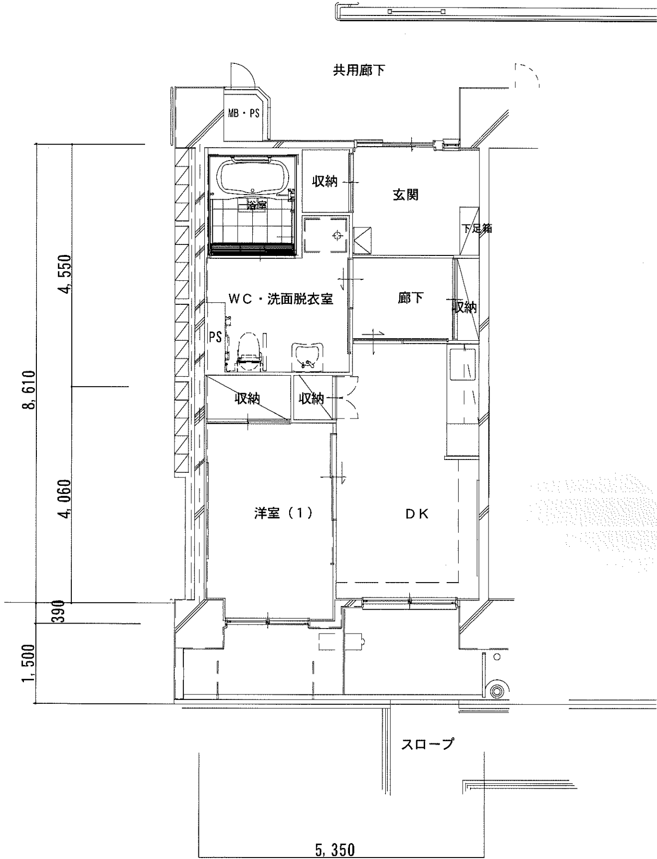
1DK車イス
