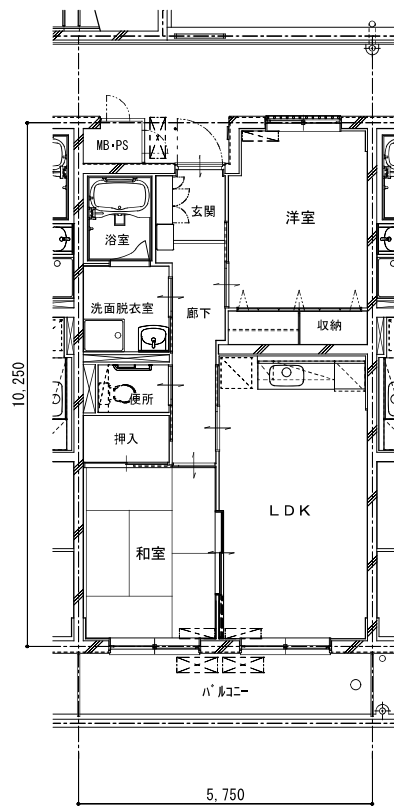
2LDK平面図
