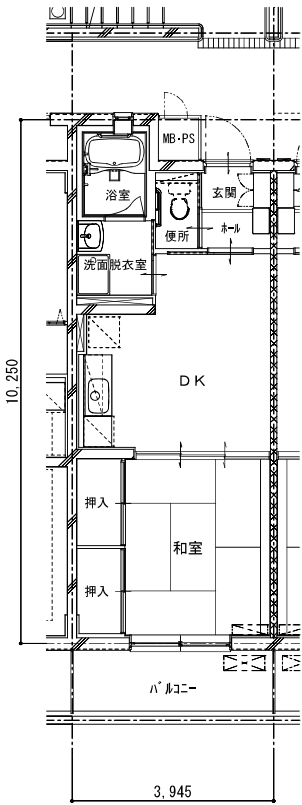
1DK平面図
