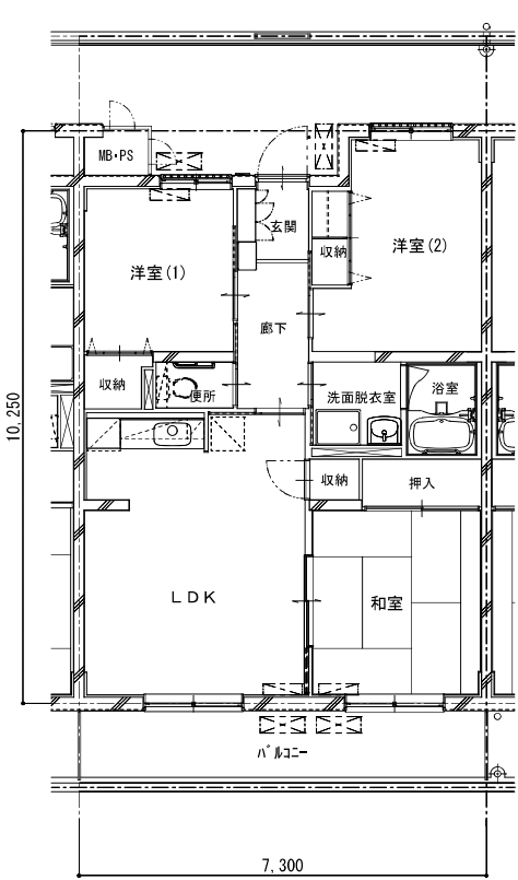
3LDK平面図
