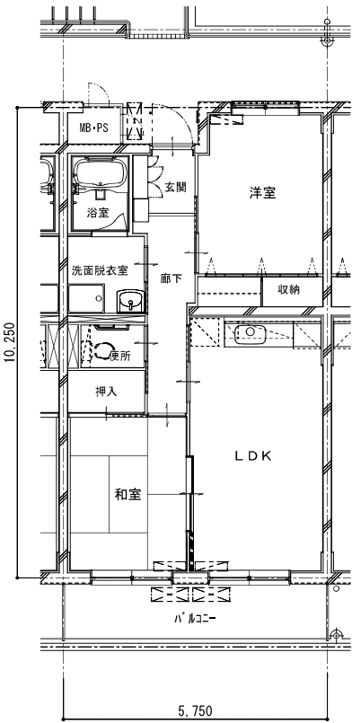
2LDK平面図
