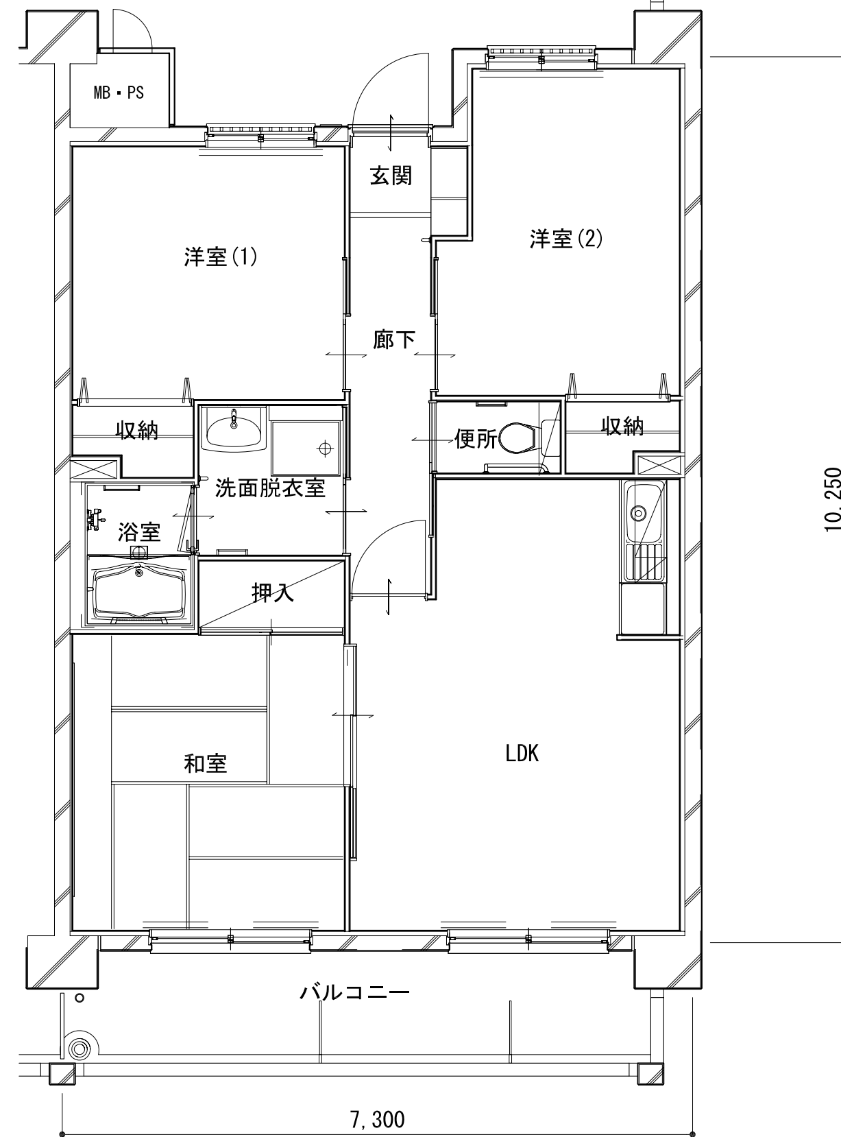
3LDK型(妻面)平面図
