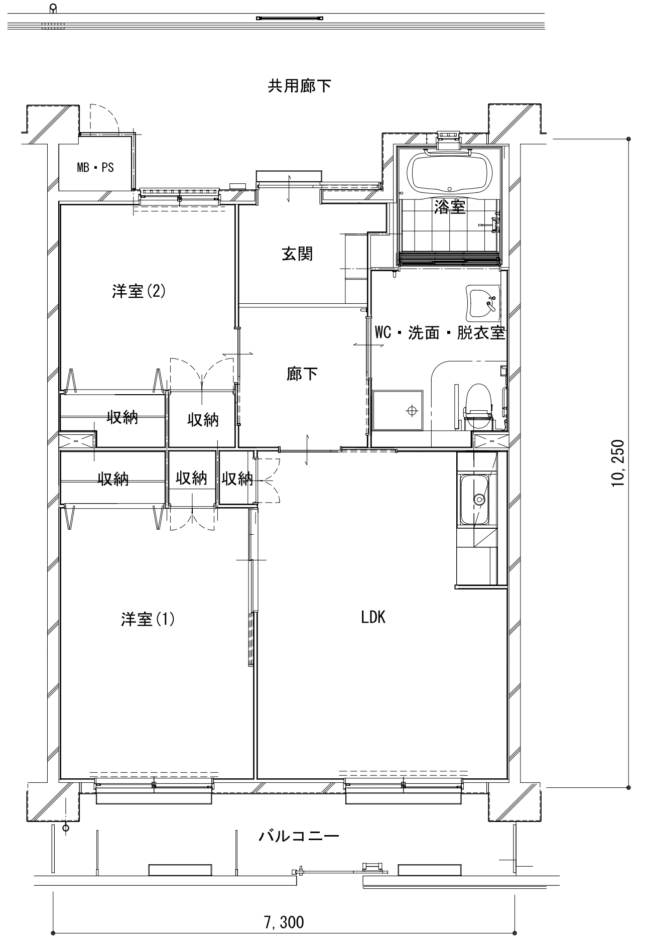
2LDK身障者型平面図
