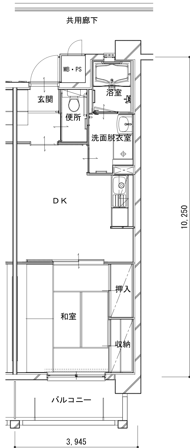
1DK型 (妻面) 平面図
