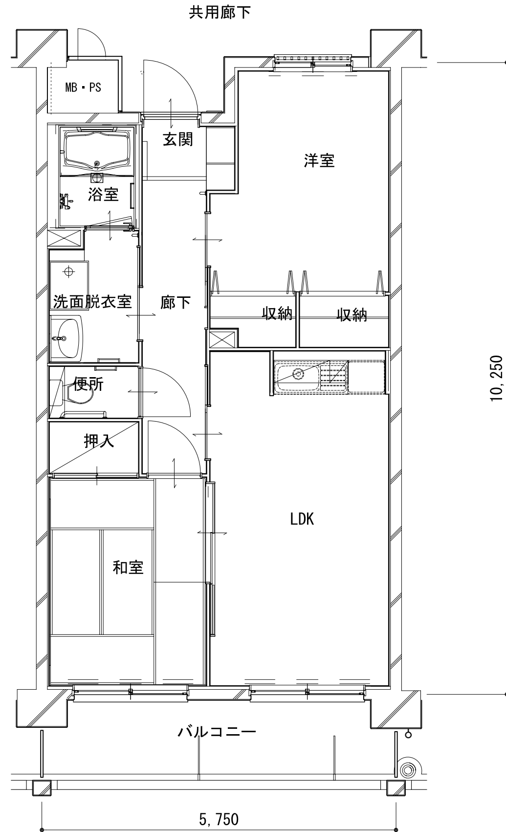
2LDK型平面図
