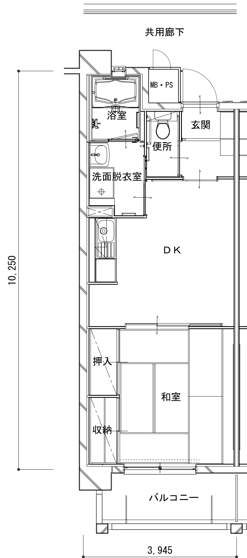
1DK型 (妻面) 平面図
