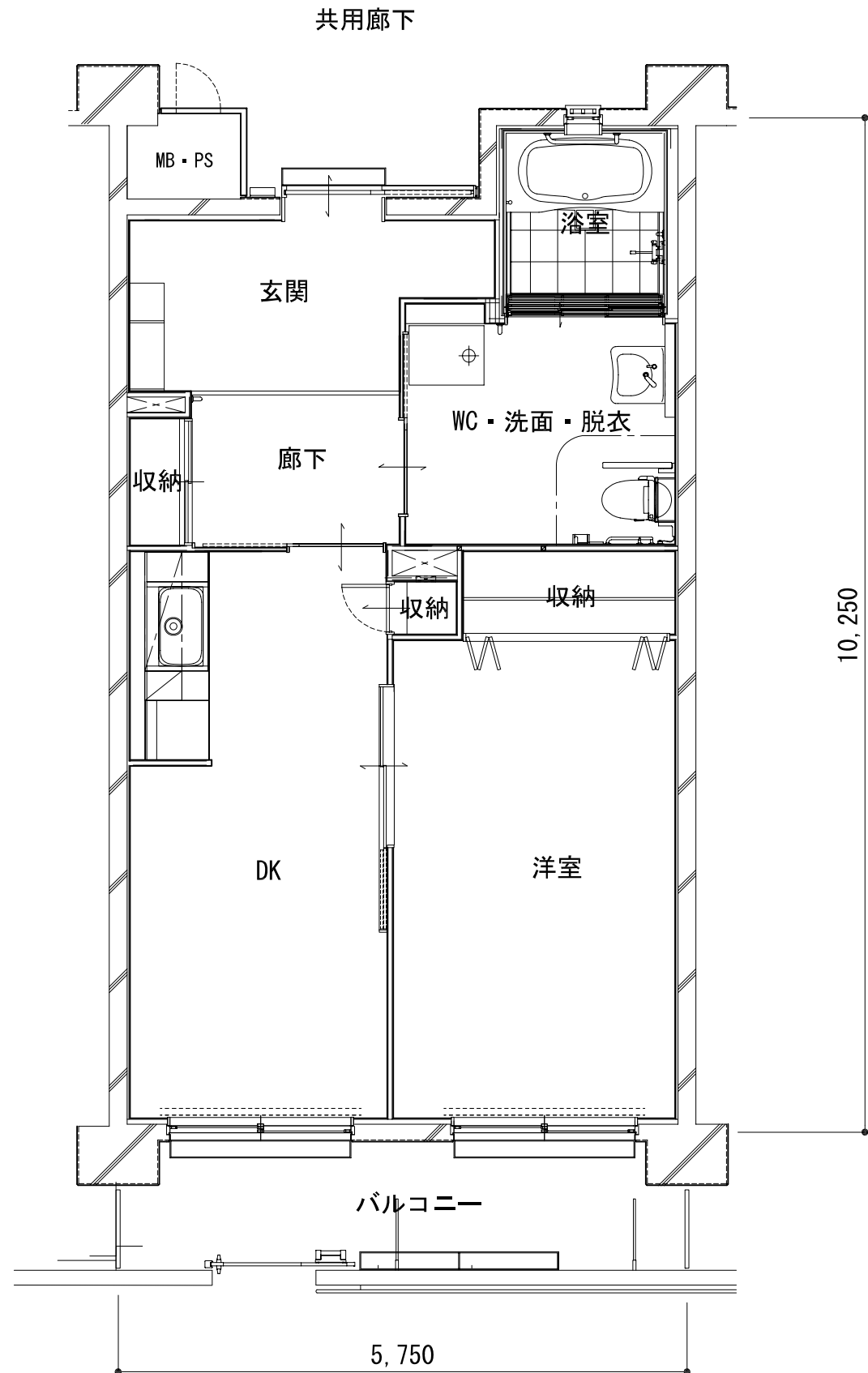
1DK身障者型平面図
