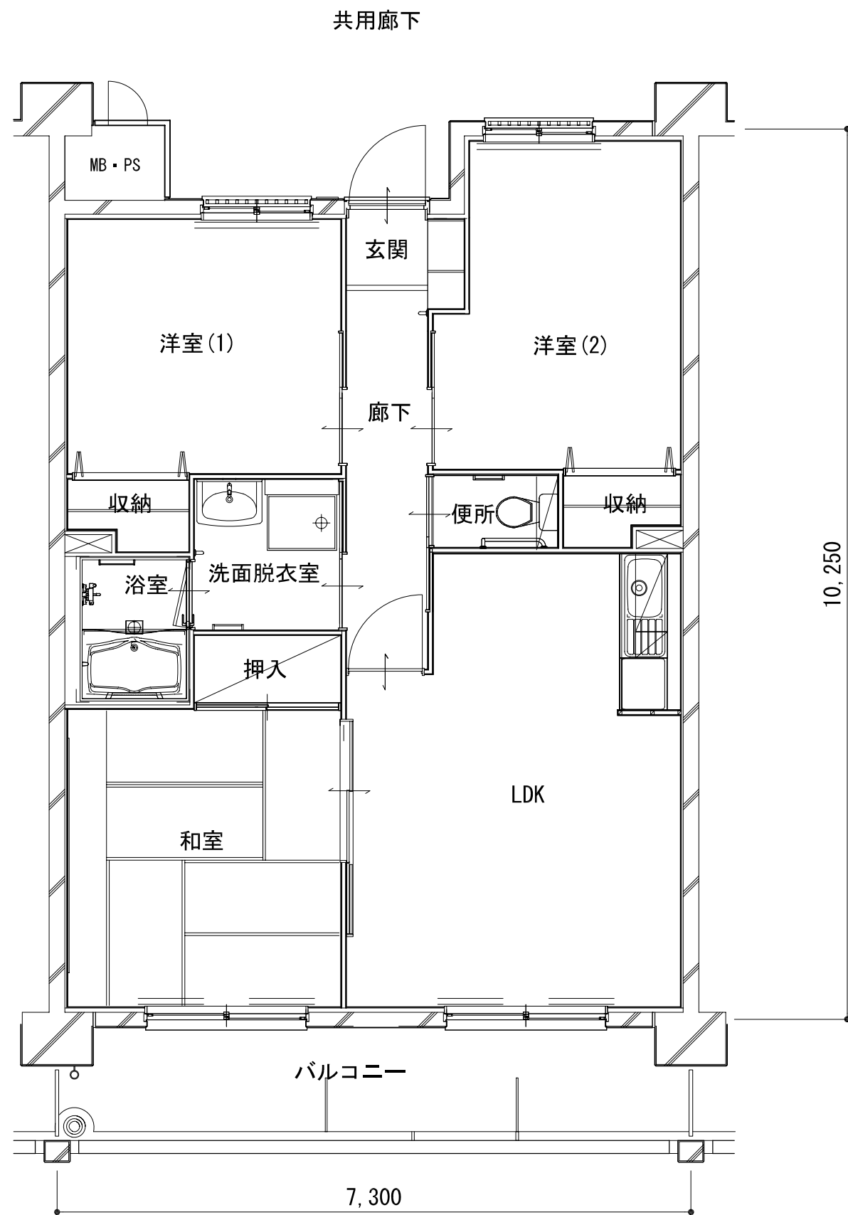
3LDK型平面図
