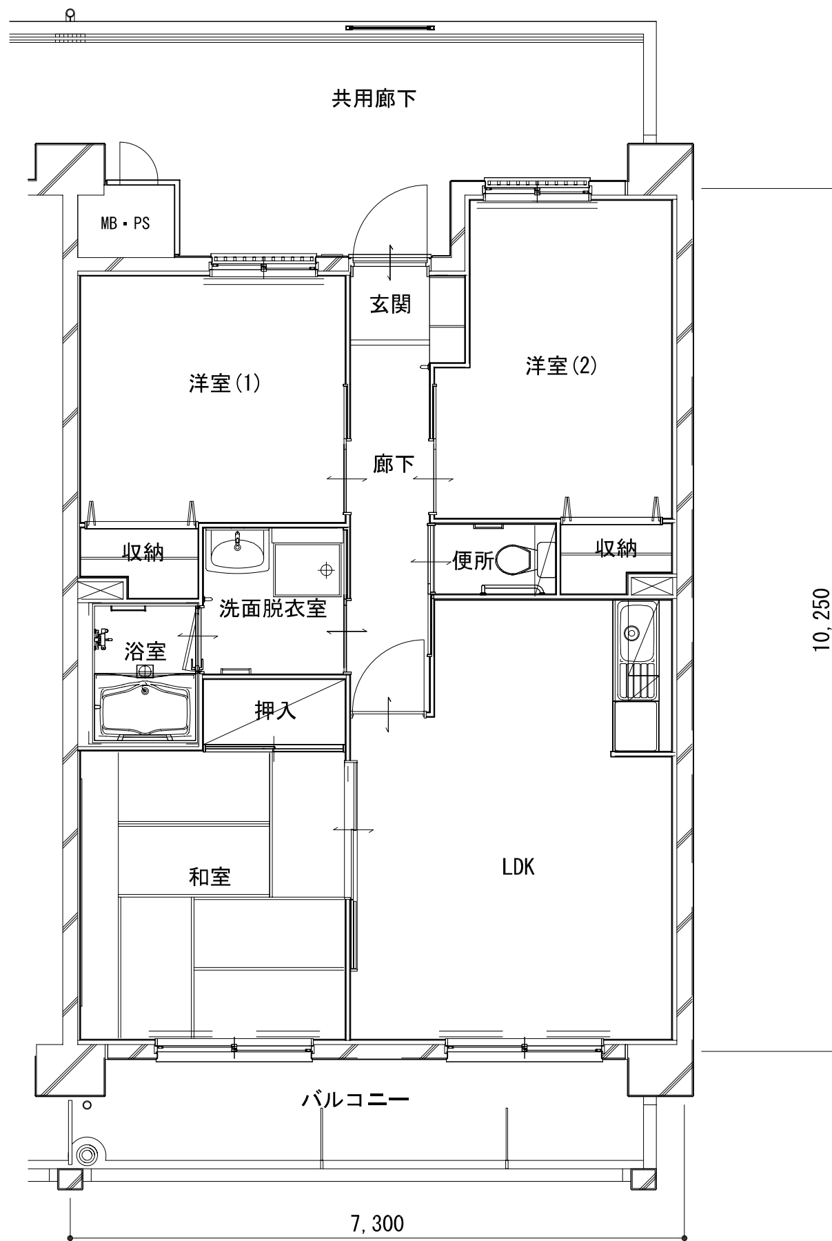
3LDK型(妻面)平面図
