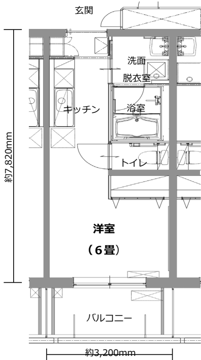
<専用住戸の間取り図>
